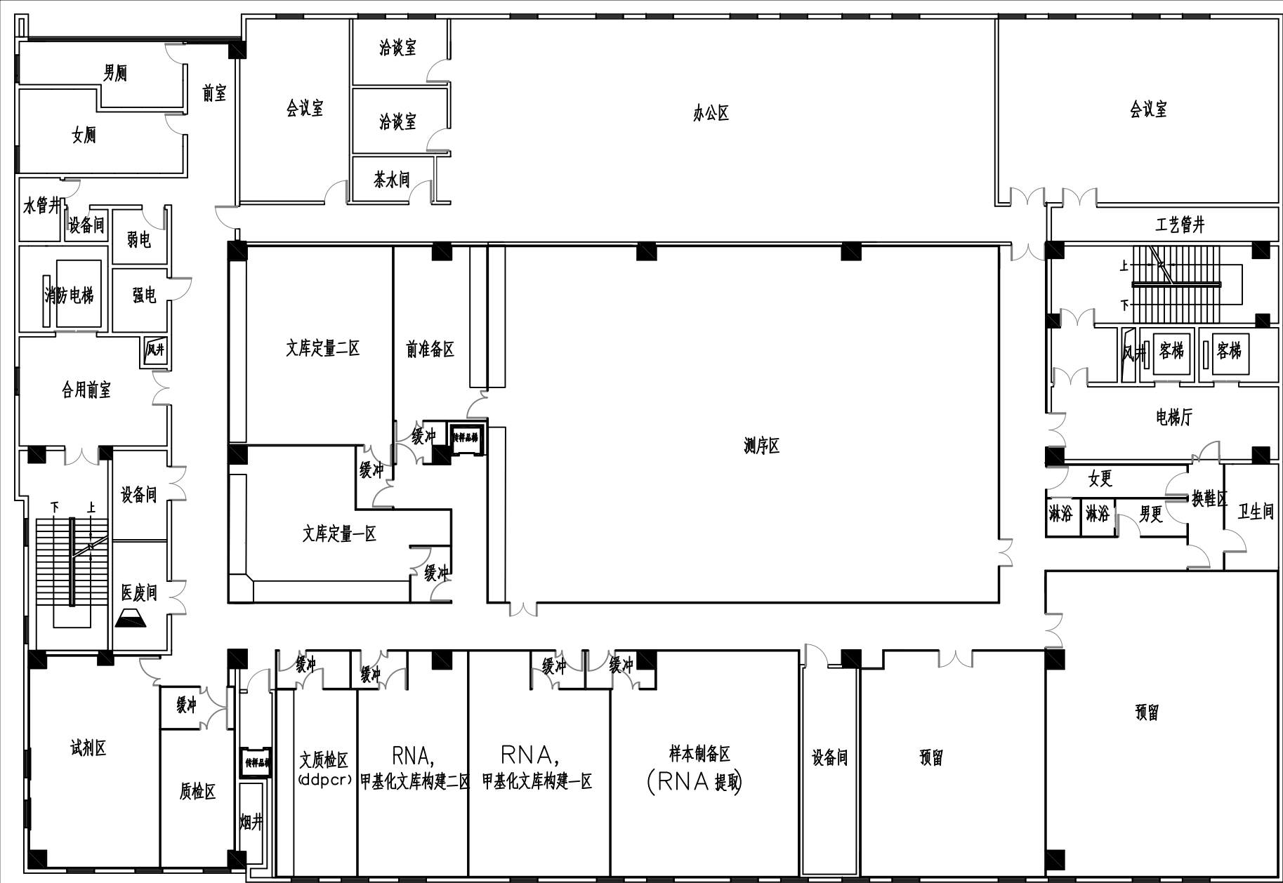
附图3-1 建设项目A栋2F平面布置图
