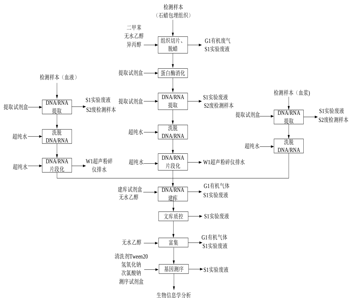
图 2-1 高通量测序工艺流程图
