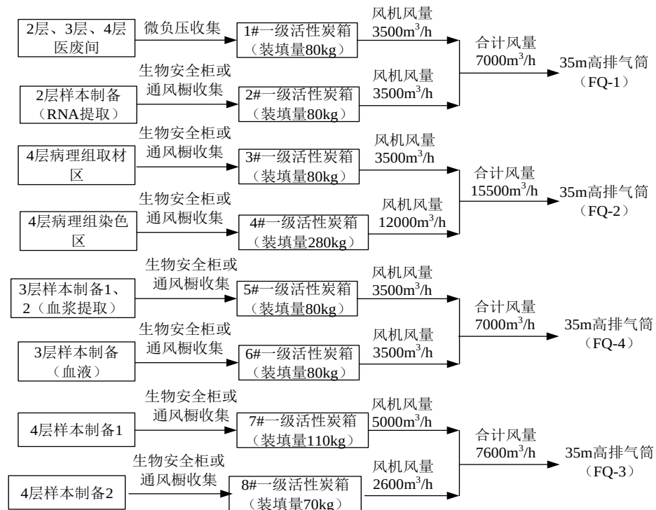
图 3.3-5 实际废气收集处理管道布置示意图
