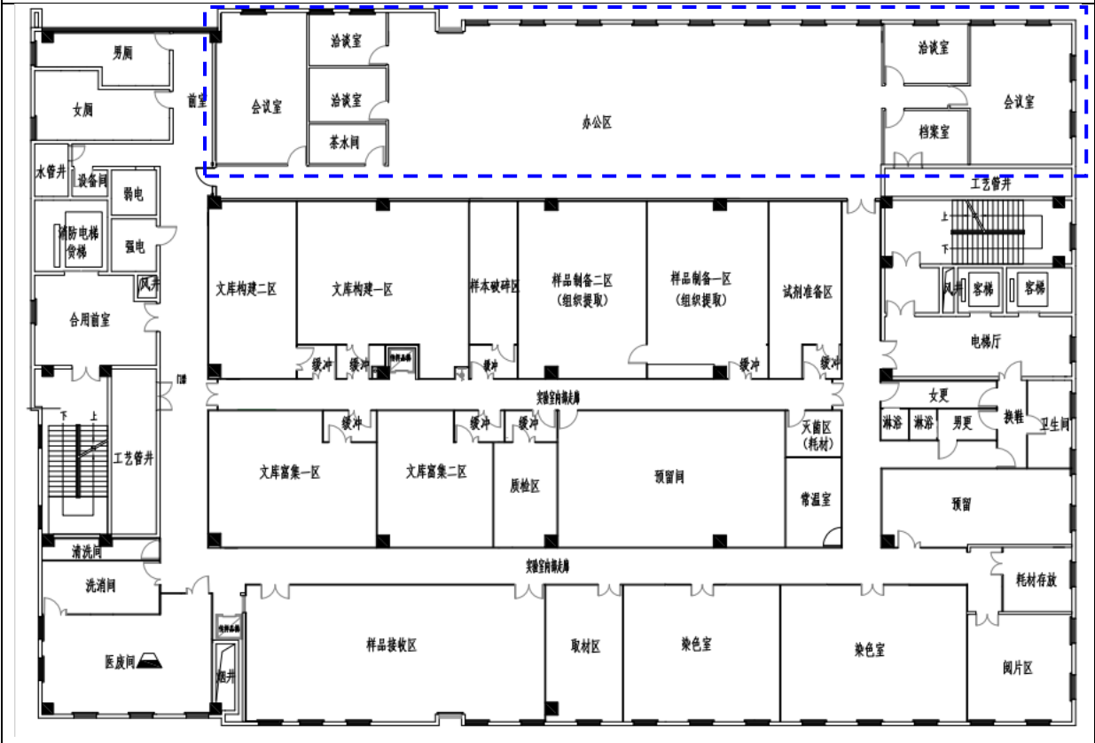
图 3.3-3b 实际建设 4F 平面布置图（虚线框为变动部分）
