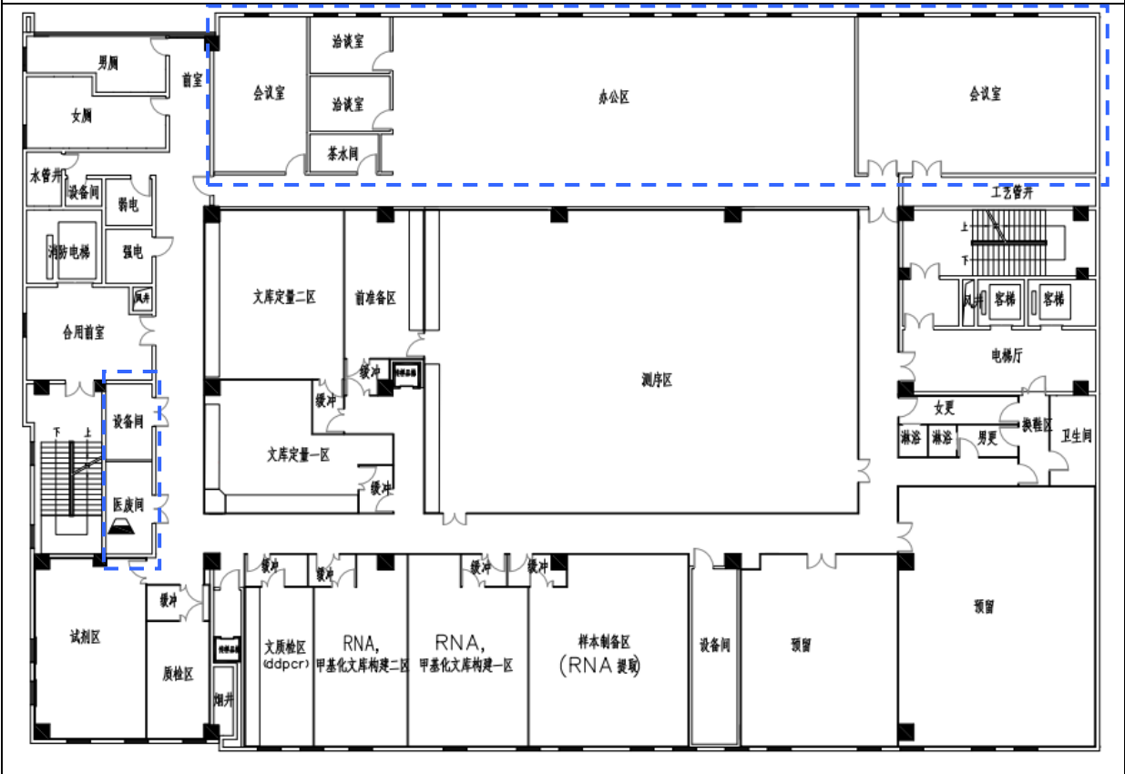
图 3.3-1b 实际建设 2F 平面布置图（虚线框为变动部分）
