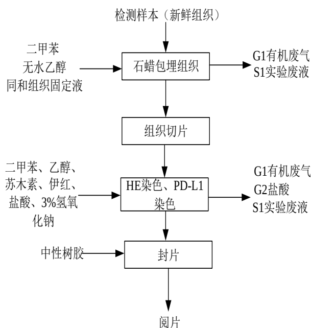
图 2-2 病理组检测工艺流程图
