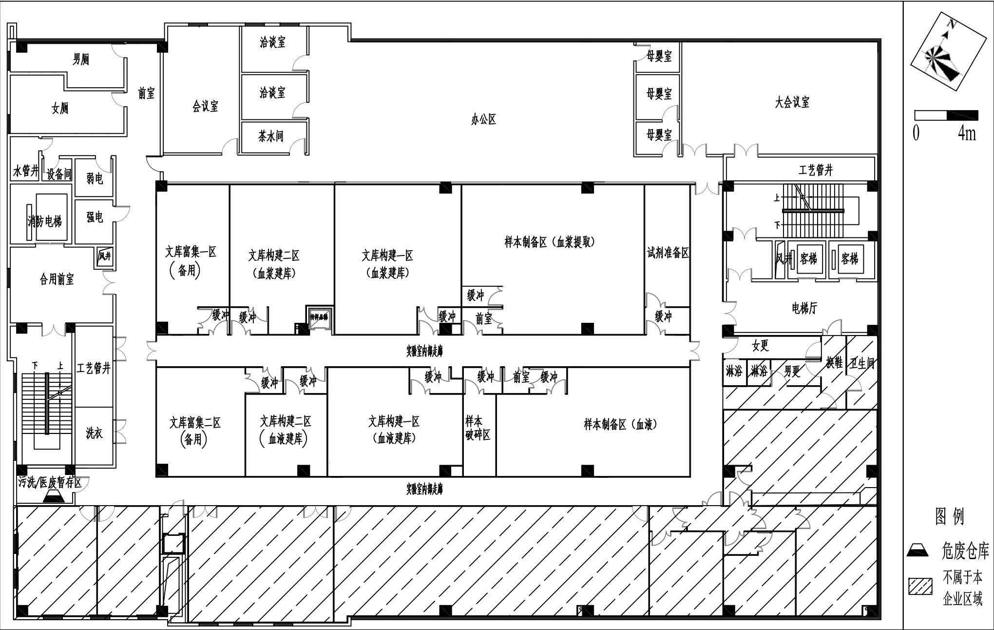
附图3-2 建设项目A栋3F平面布置图
