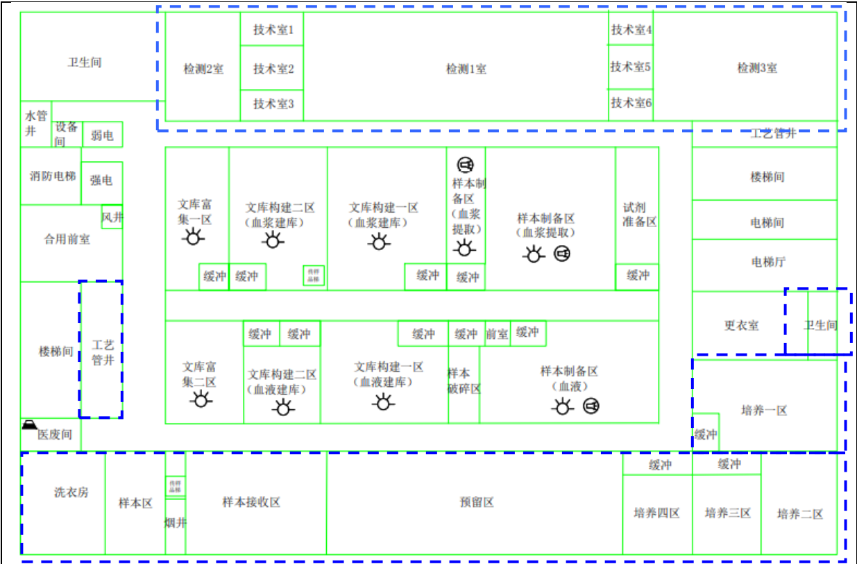
图 3.3-2a 原环评中 3F 平面布置图（虚线框为变动部分）
