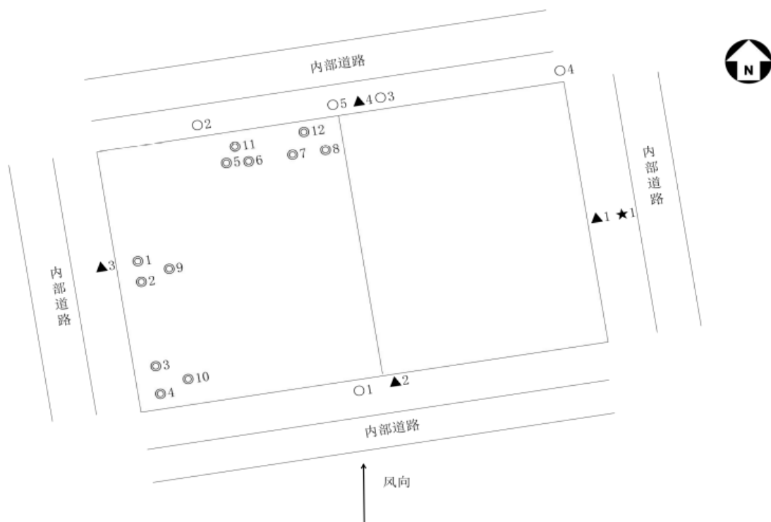
图 3-6 废气、废水和噪声监测点位示意图（2022.4.28、2022.4.29）
