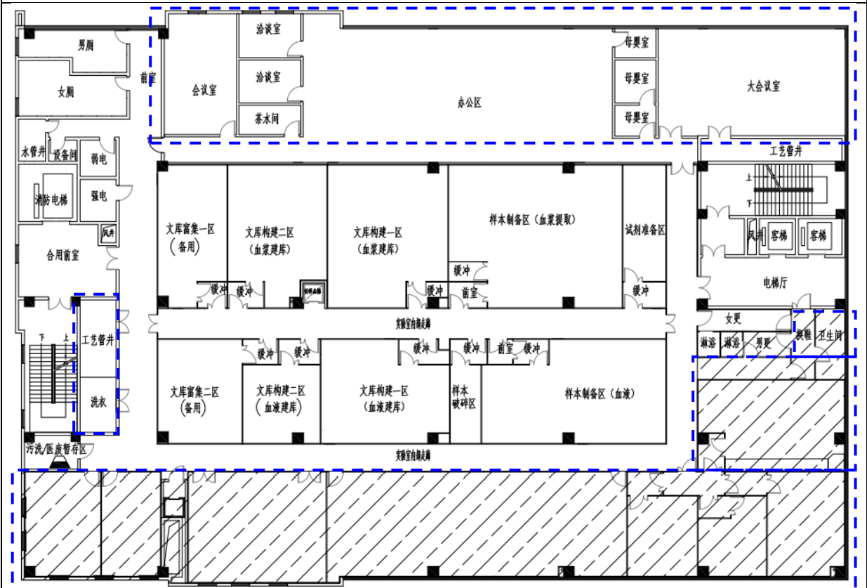
图 3.3-2b 实际建设 3F 平面布置图（虚线框为变动部分，阴影部分为其他企业）
