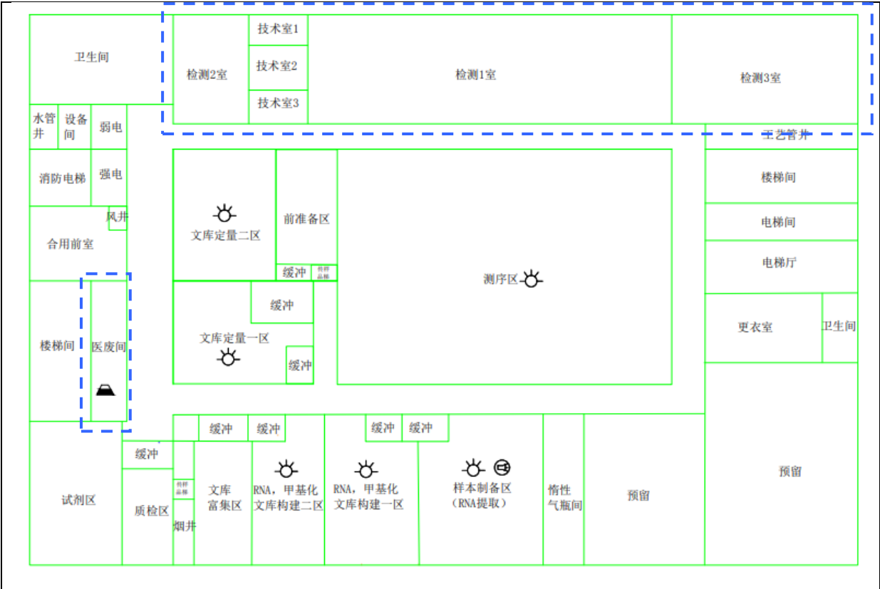
图 3.3-1a 原环评中 2F 平面布置图（虚线框为变动部分）
