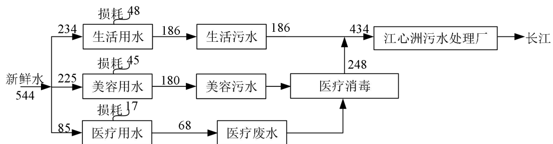
图 2-2 项目建成后全院水平衡图 (t/a)
