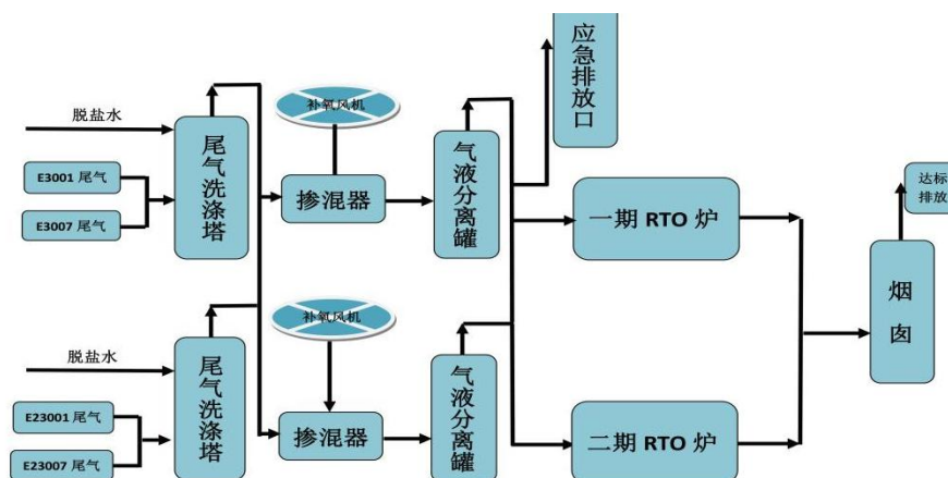
图 2-3 本项目 RTO 废气处理工艺流程图
