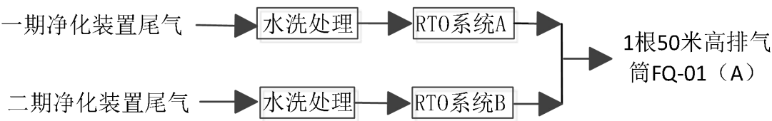
图 2-2 本项目建成后废气治理情况
