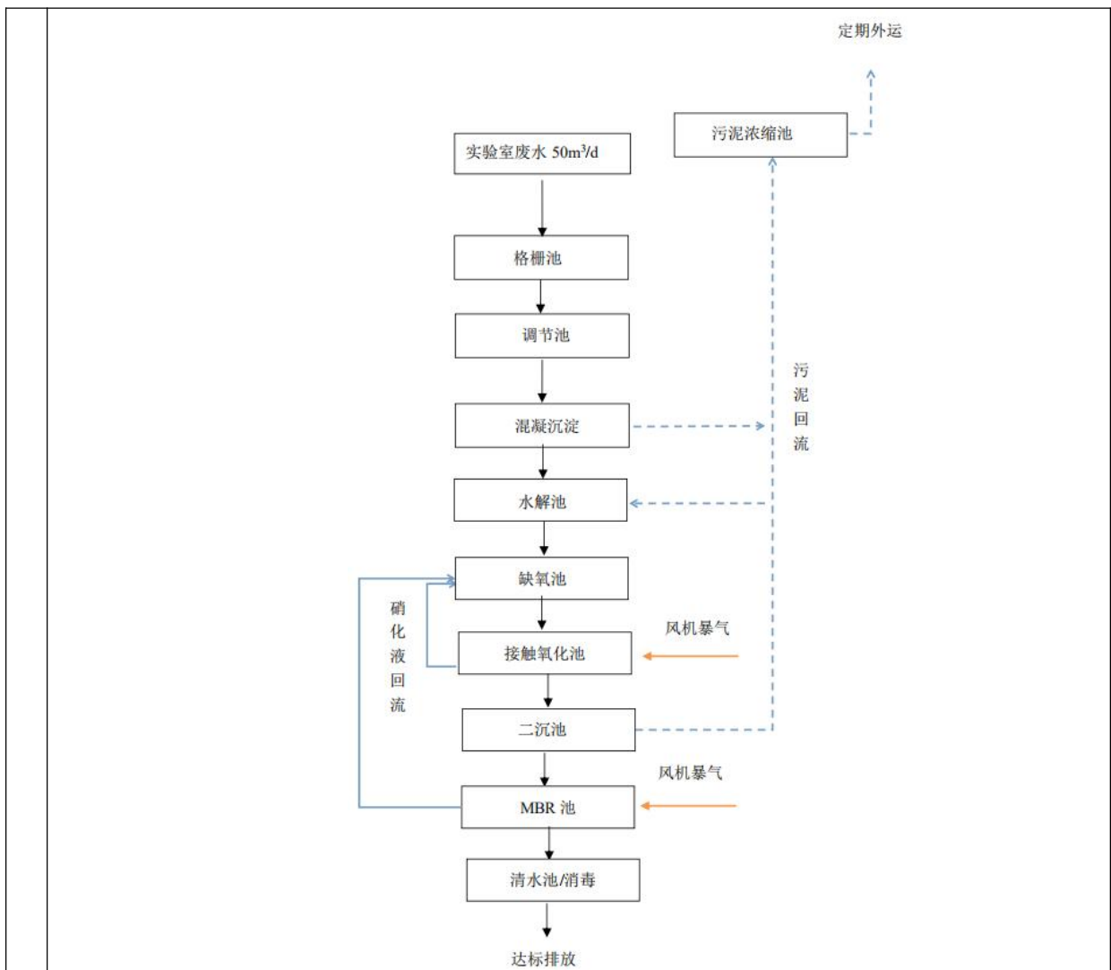
图 4-1 慧科现有污水处理站废水处理工艺流程图
