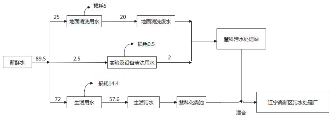
图 2-1 水平衡图 单位 m^3/a
